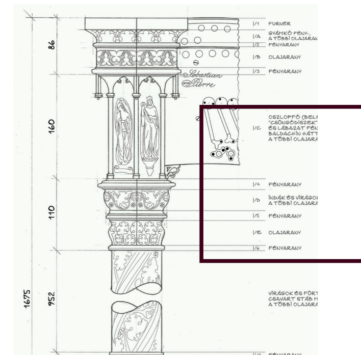
■ Az oszlop vetületi rajza
